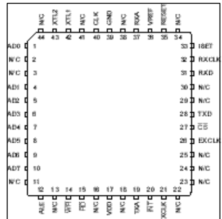
44-Lead TQFP 73K222AL-IGT
