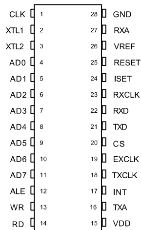
600-Mil 28-Pin DIP 73K222AL-IP
