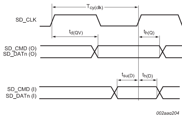
Fig 27. SD/MMC timing
